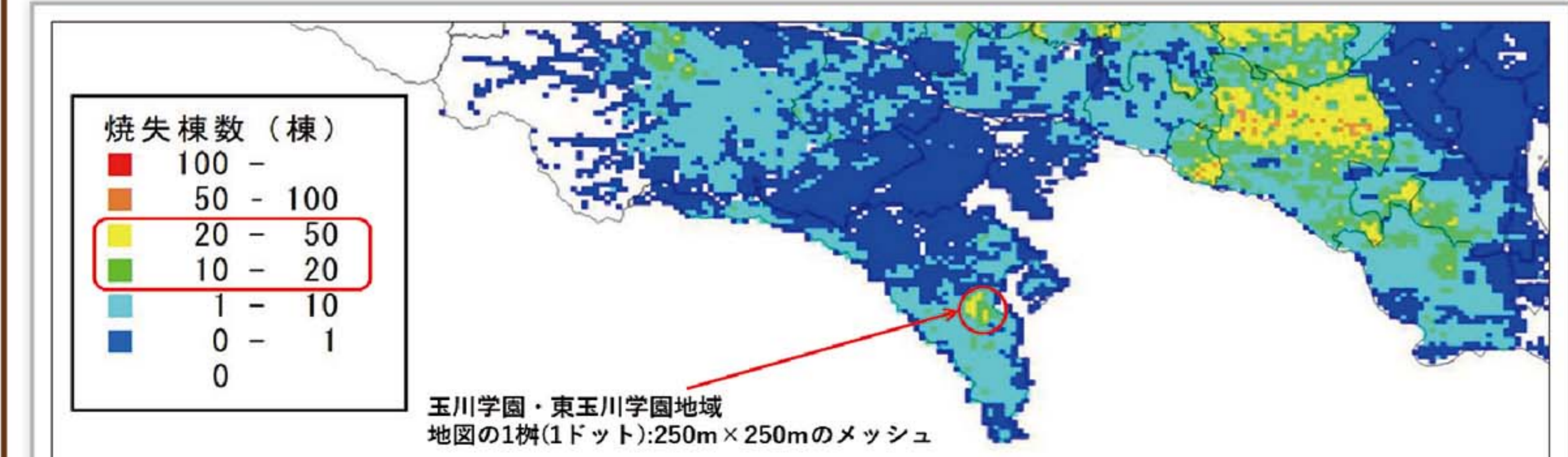
図 焼失棟数分布(多摩東部直下地震、冬・夕方、風速8m/s)
