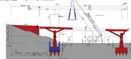
デッキ橋桁設置工事の計画図
